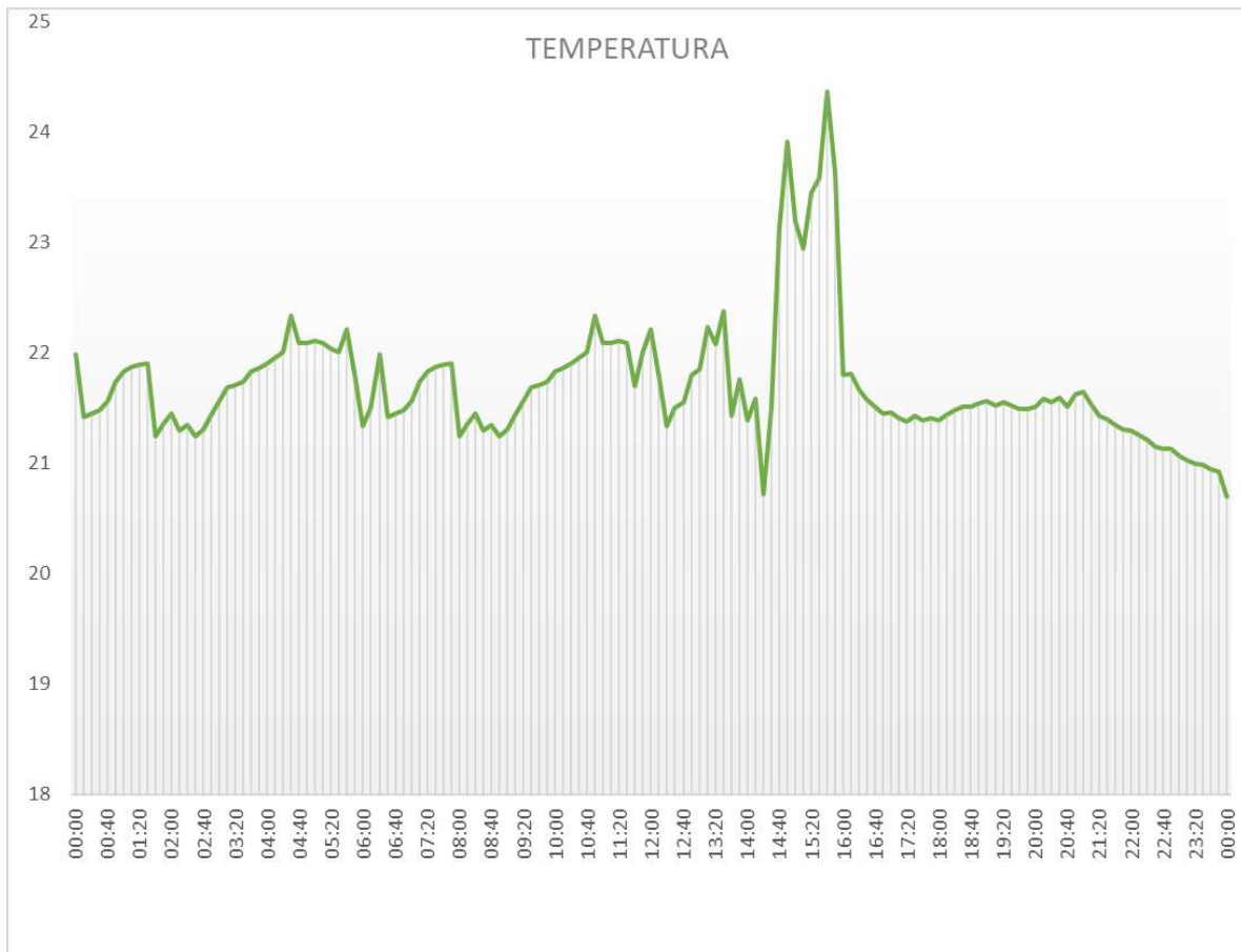
Grafica de medición temperatura
